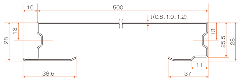
■断面図
