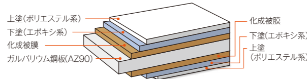
■構成図
