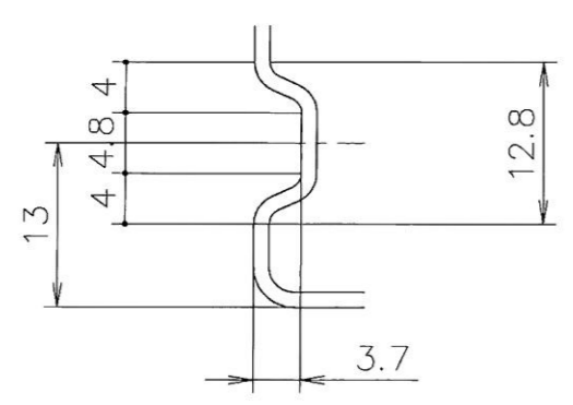
リブ詳細 (S=3/1)
