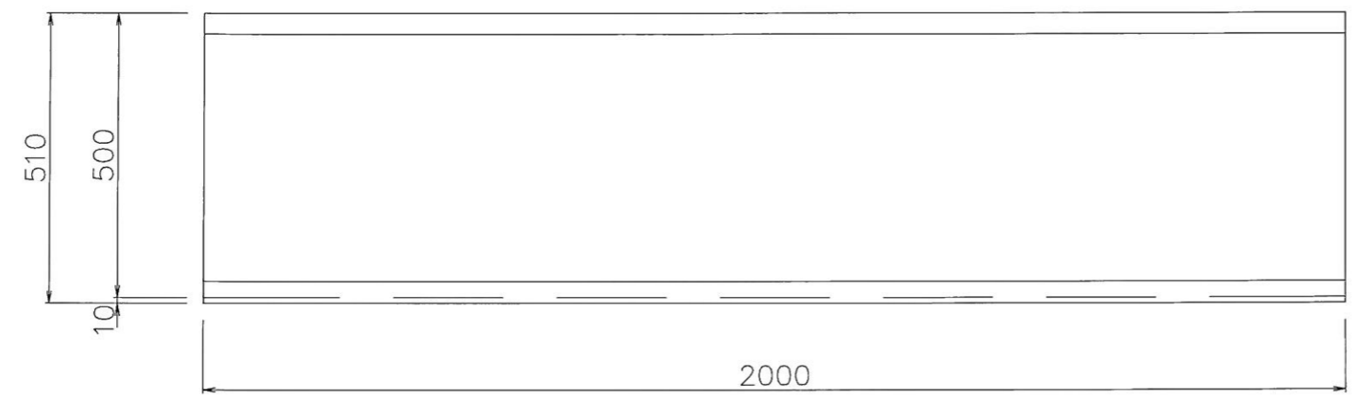
全景図 (S=1/6)
