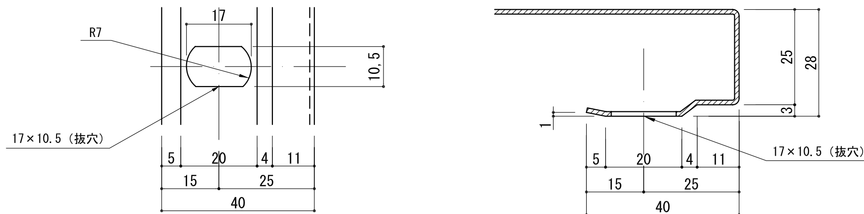
A部断面詳細 (S=1/1)
