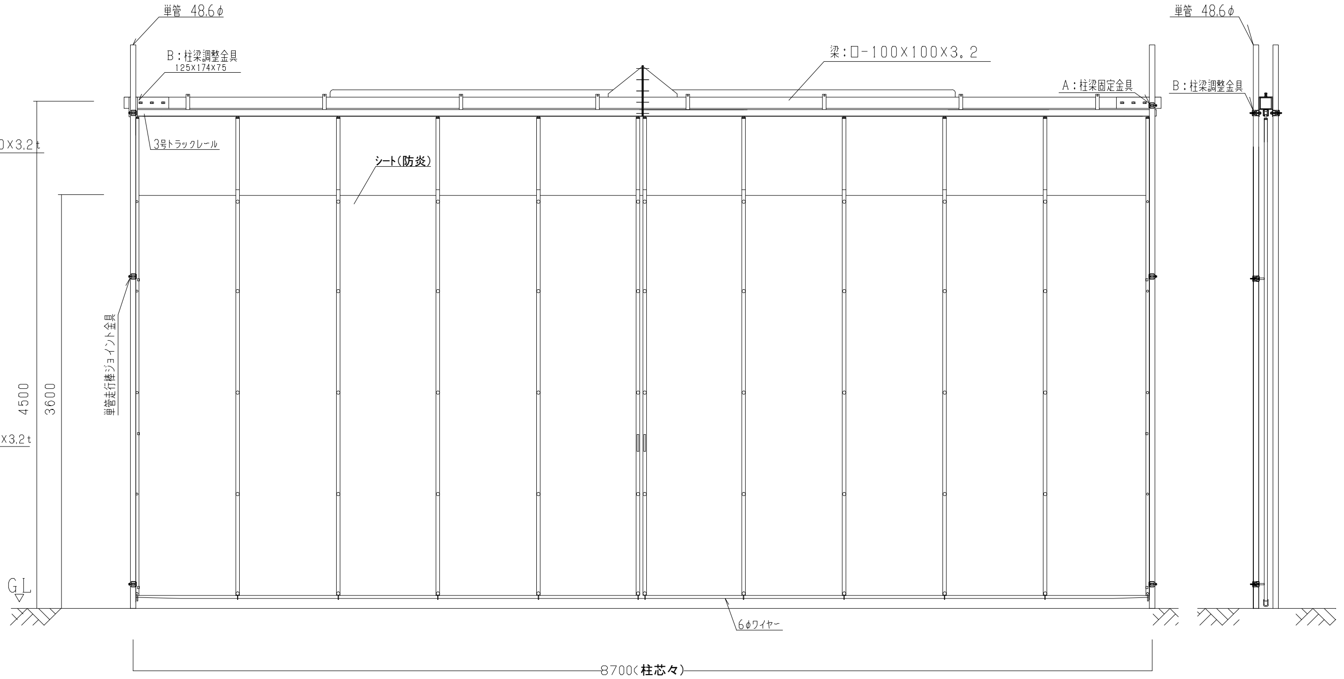
側面図
