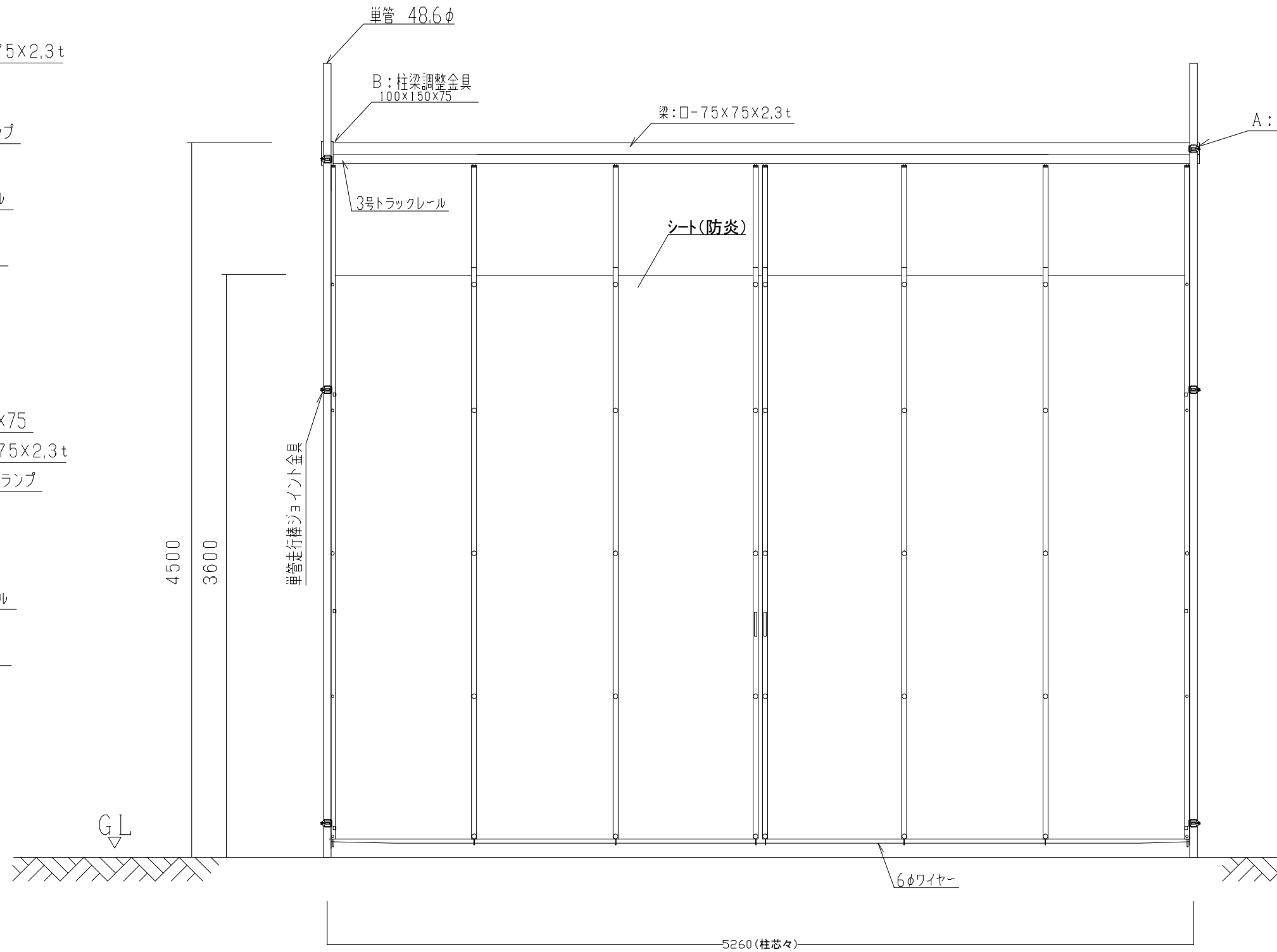
立面図
