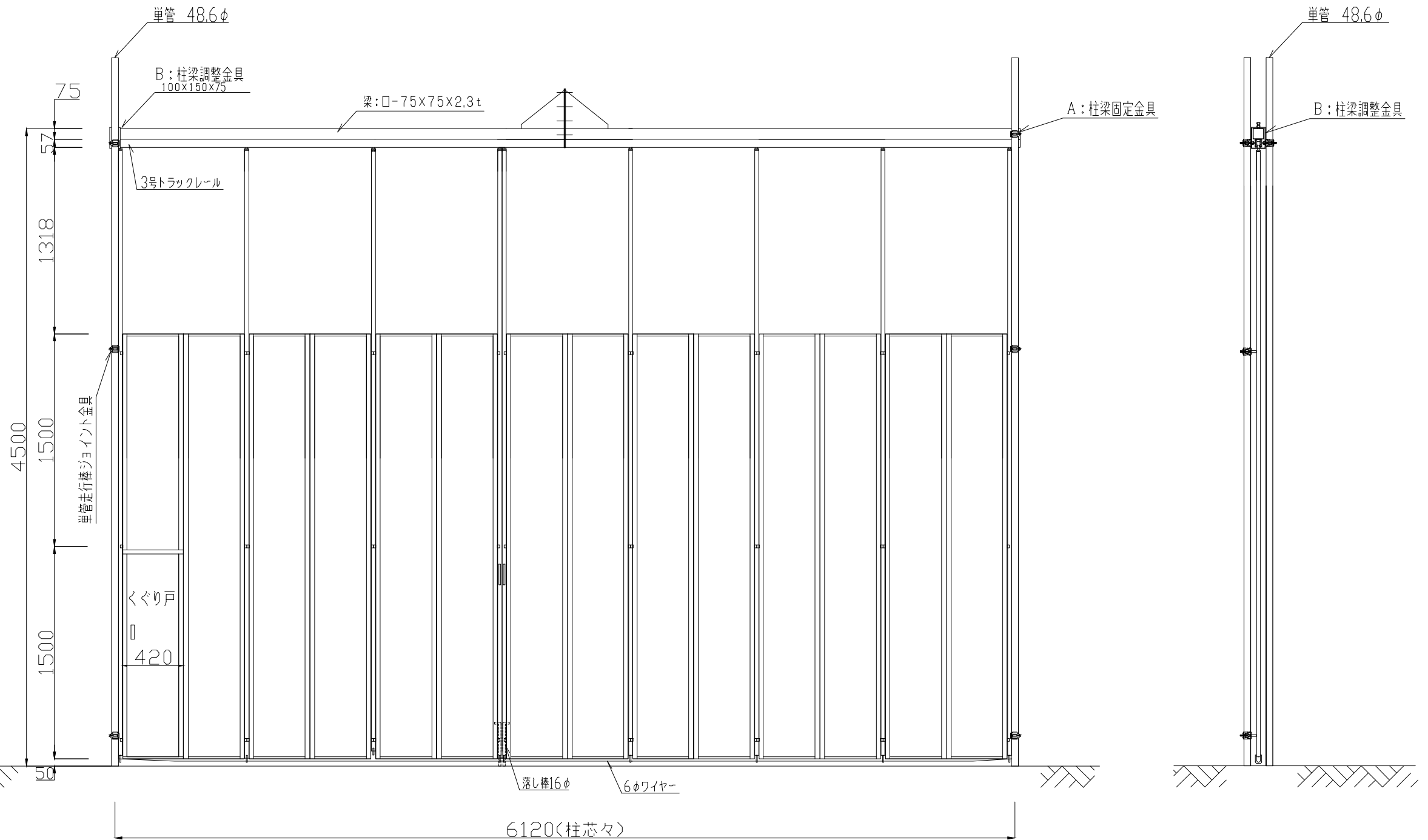
側面図
