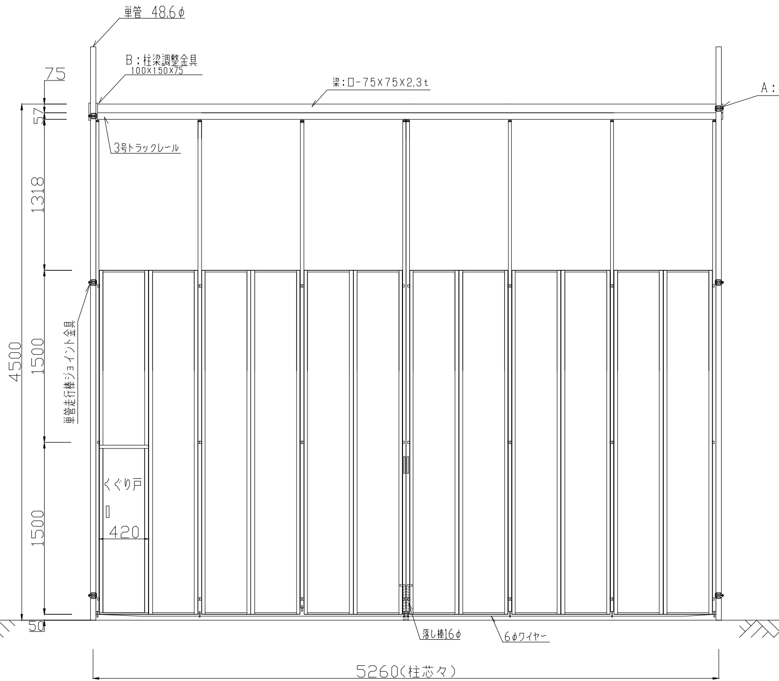
立面図
