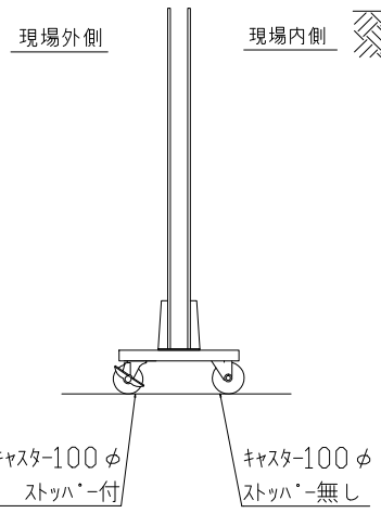
中間脚 詳細
