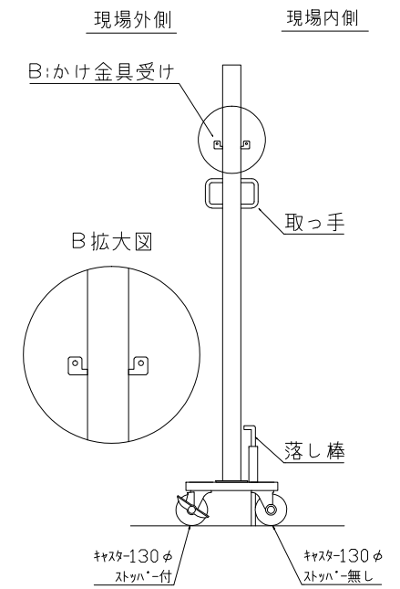
中央支柱左 詳細
