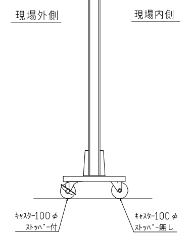
キャスタ台詳細
