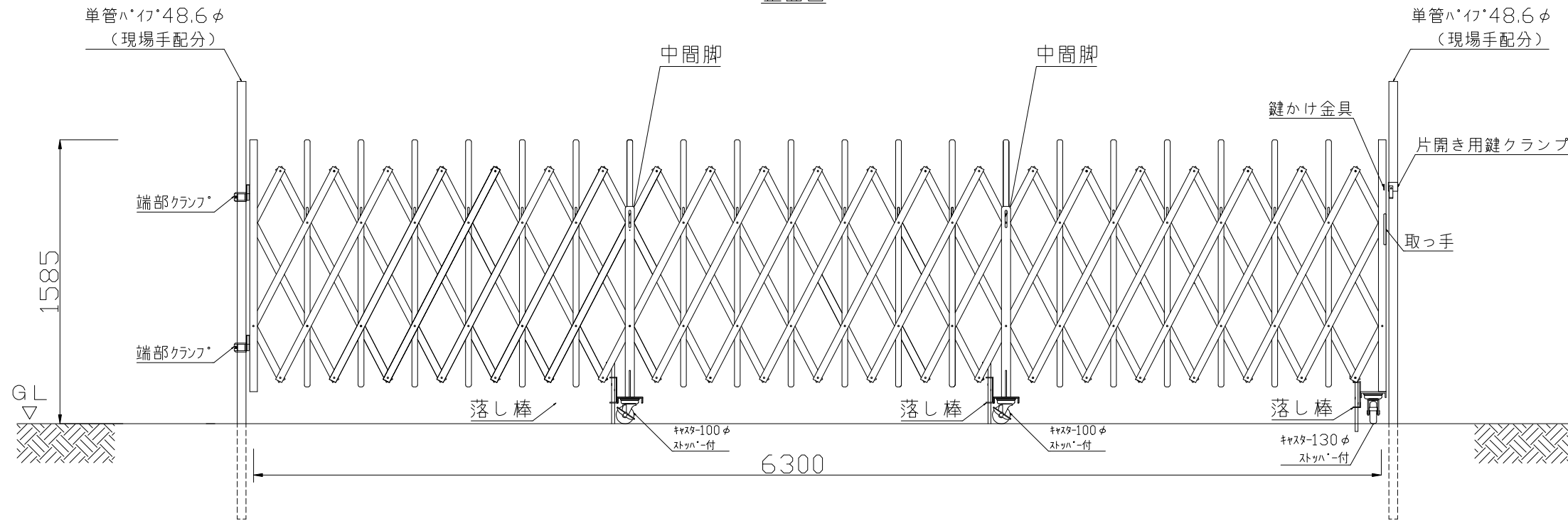
正面図
