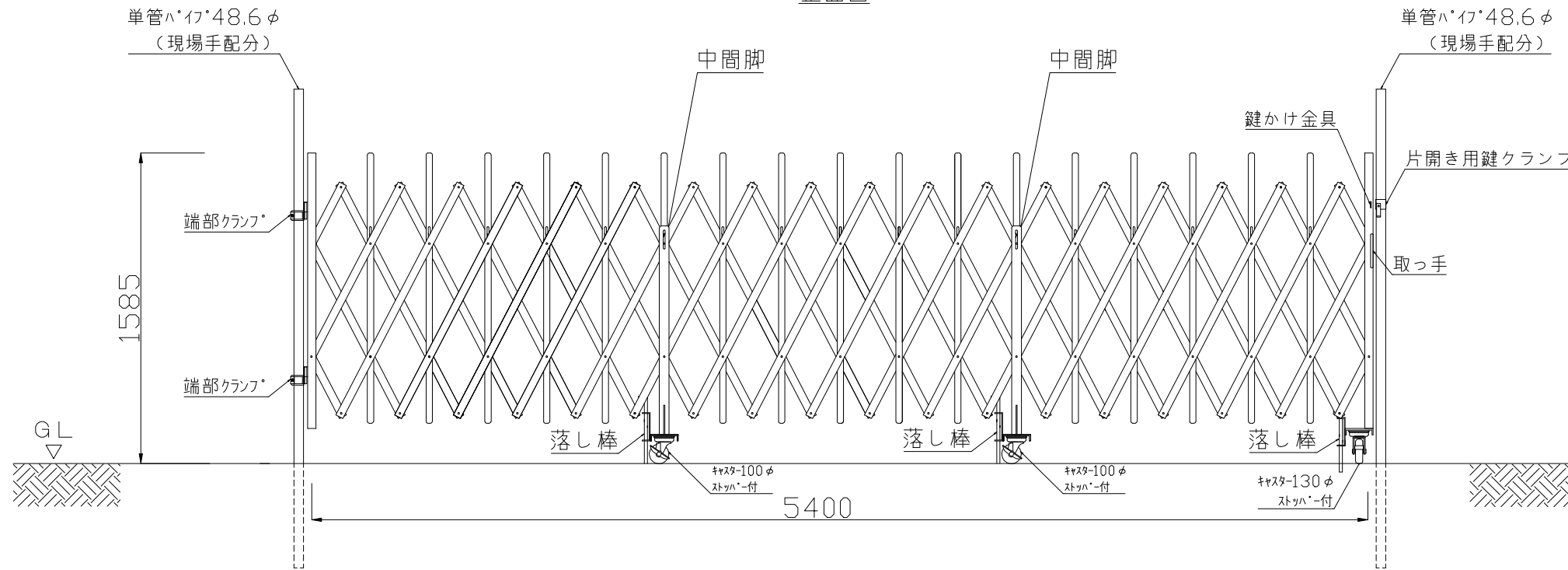
正面図
