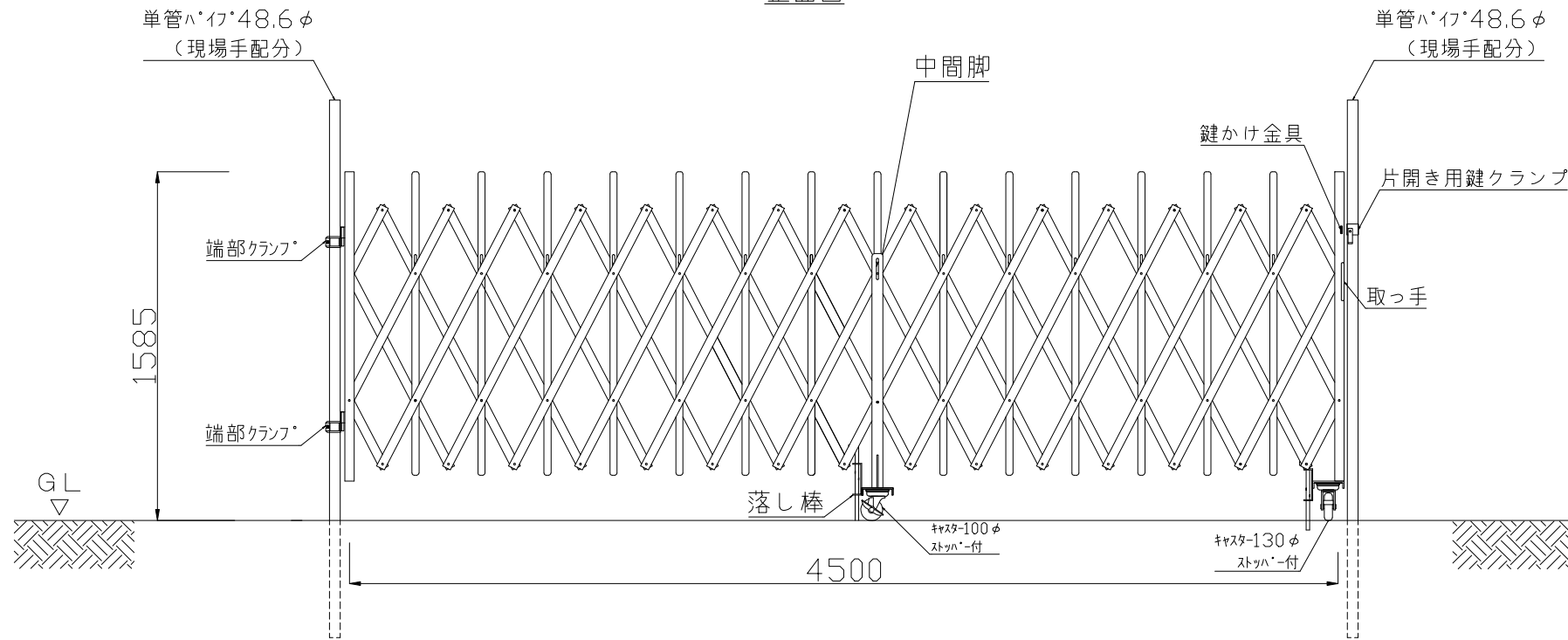
正面図
