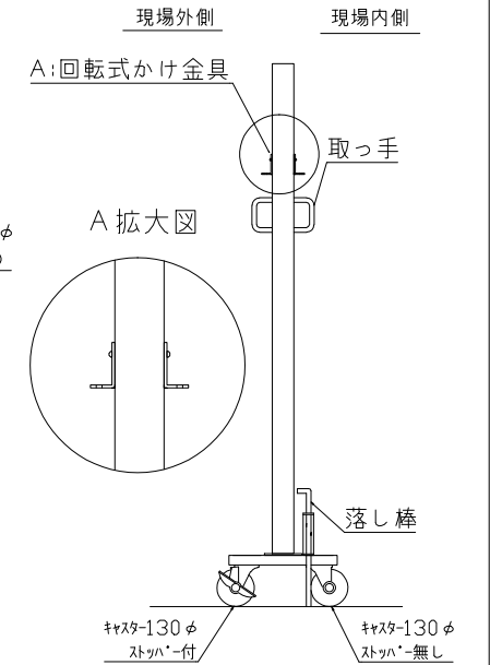
中央支柱右 詳細
