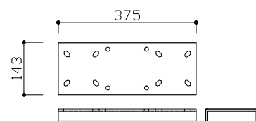
キャスタ-台詳細
