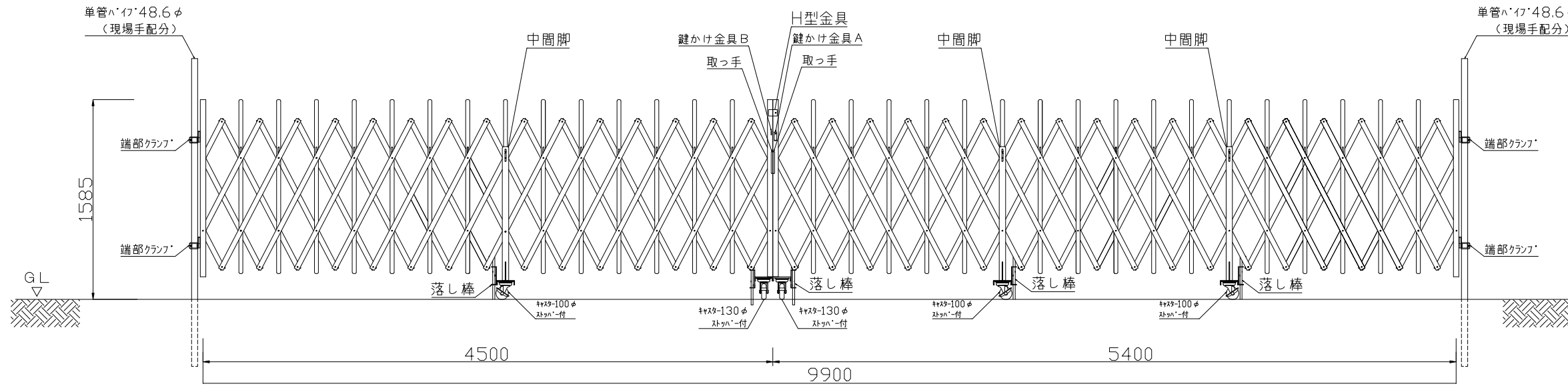
背面図
