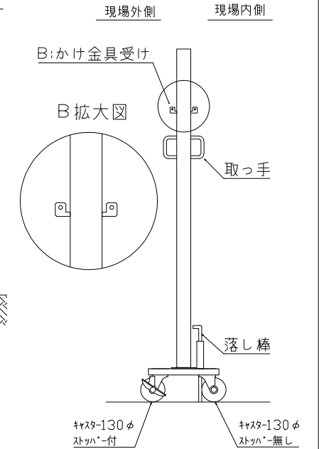
中央支柱左 詳細
