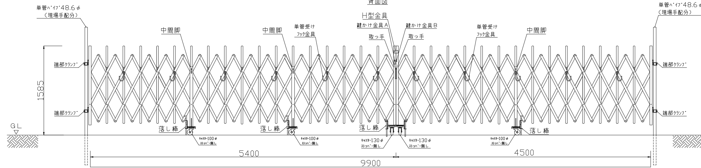
背面図
