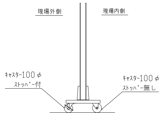
中間脚 詳細
