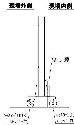
中間脚詳細
