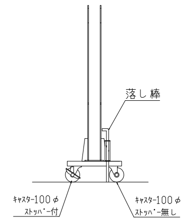
中央支柱左 詳細
