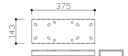
キャスター台詳細
