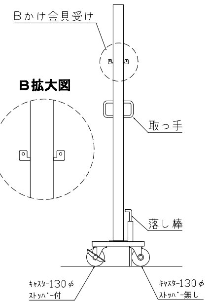
キャスター台詳細
