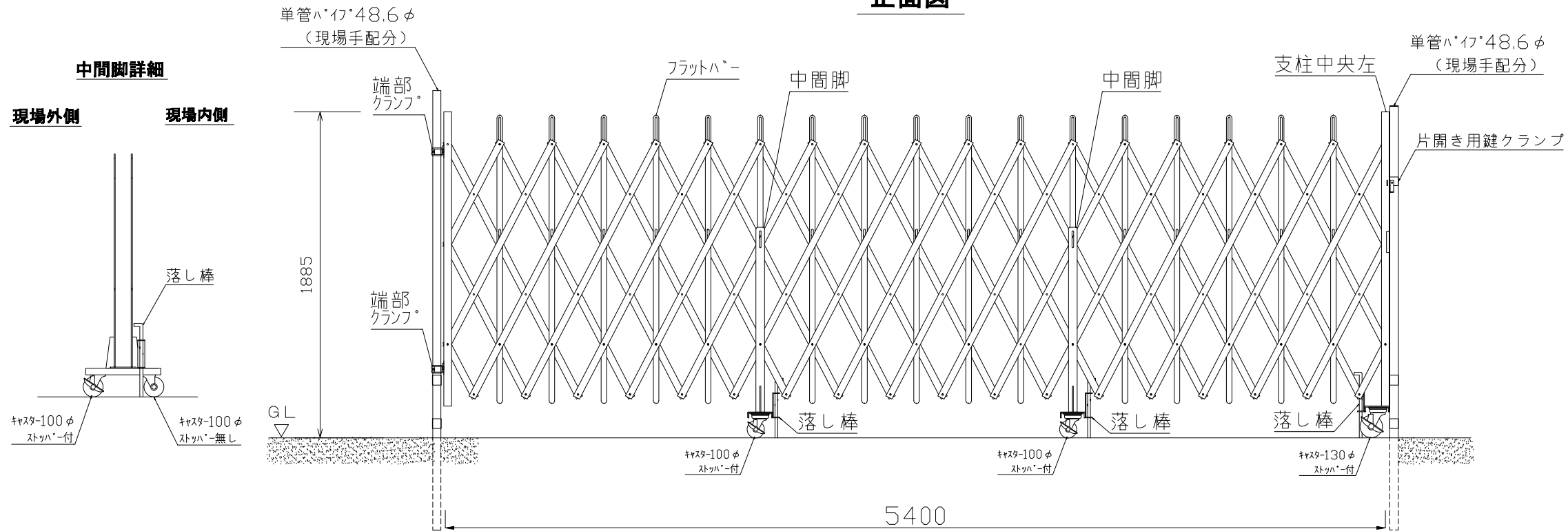
正面図
