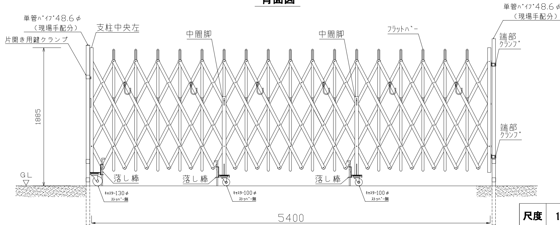
背面図
