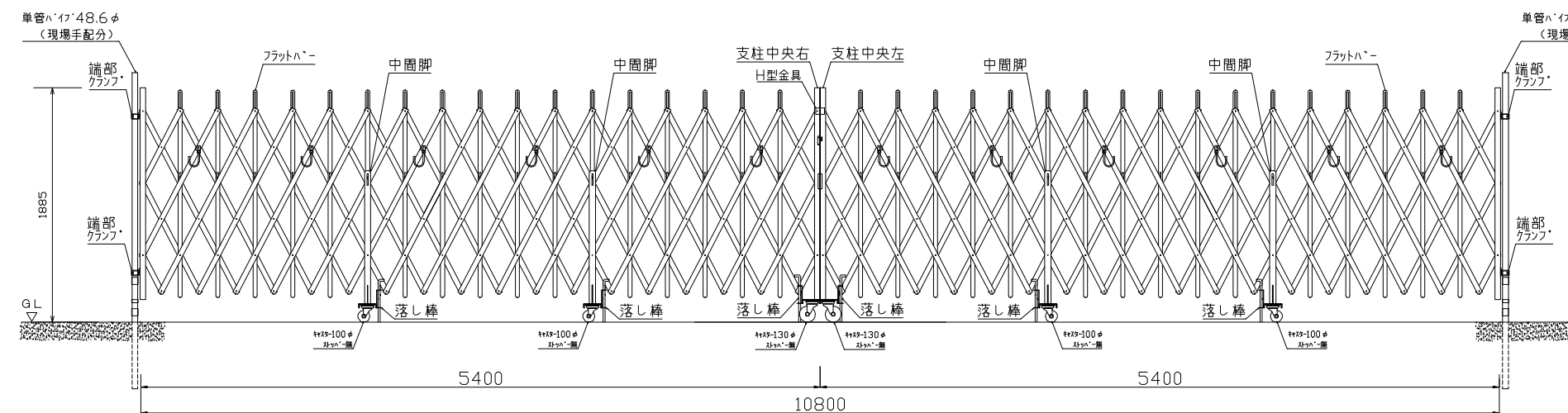
背面図
