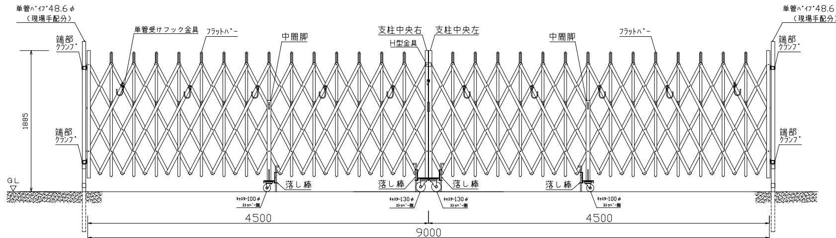
背面図
