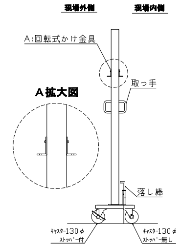
中央支柱右 詳細
