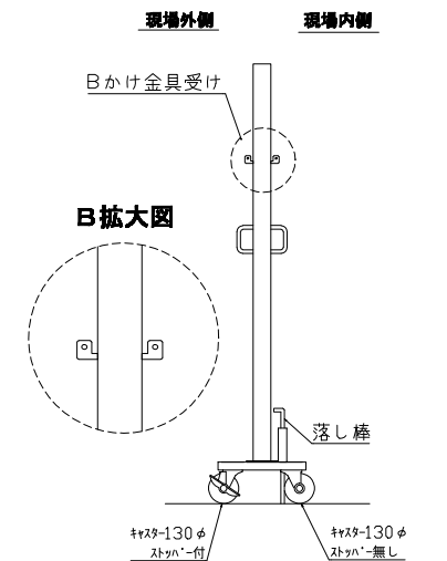
中央支柱左 詳細
