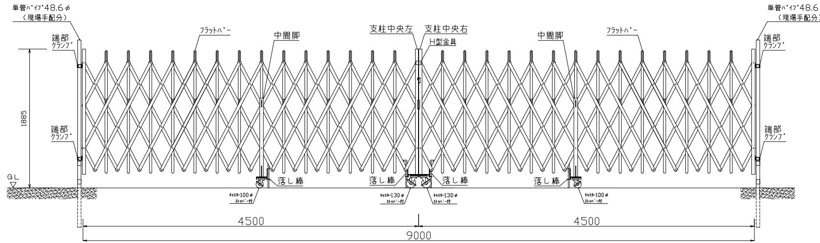
正面図
