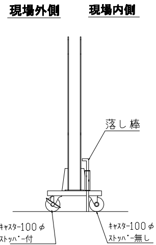
中間脚詳細
