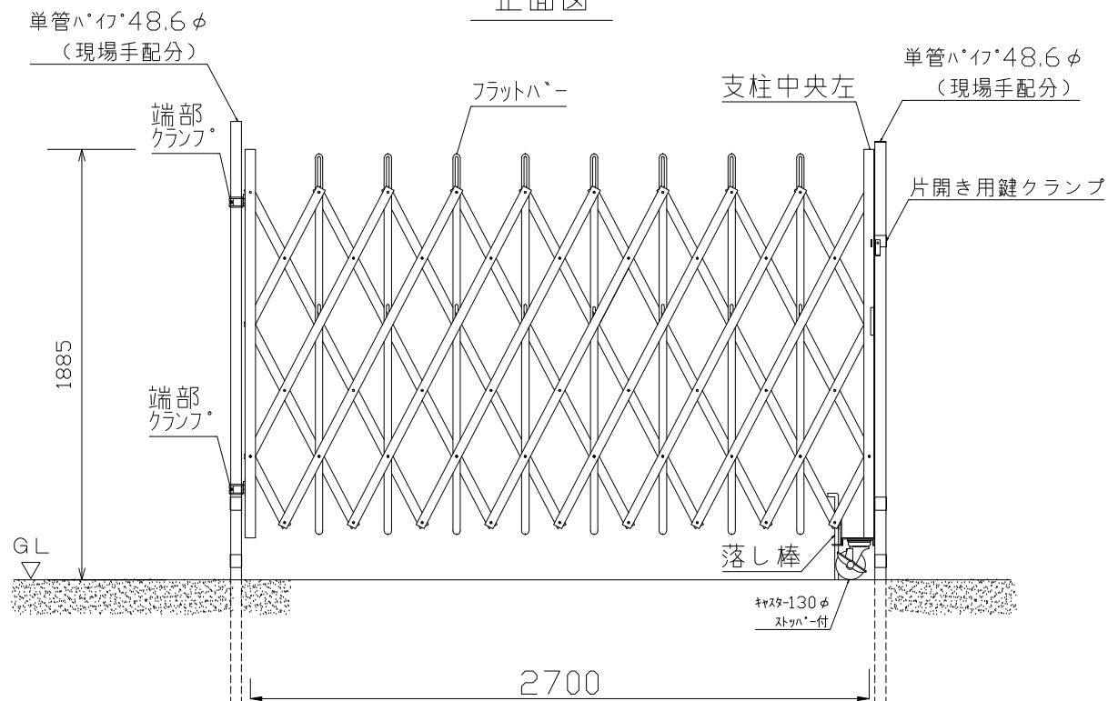
正面図
