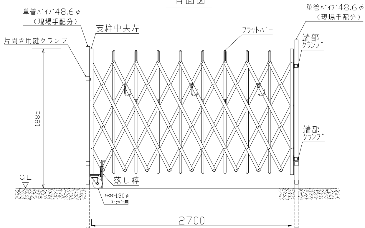
背面図
