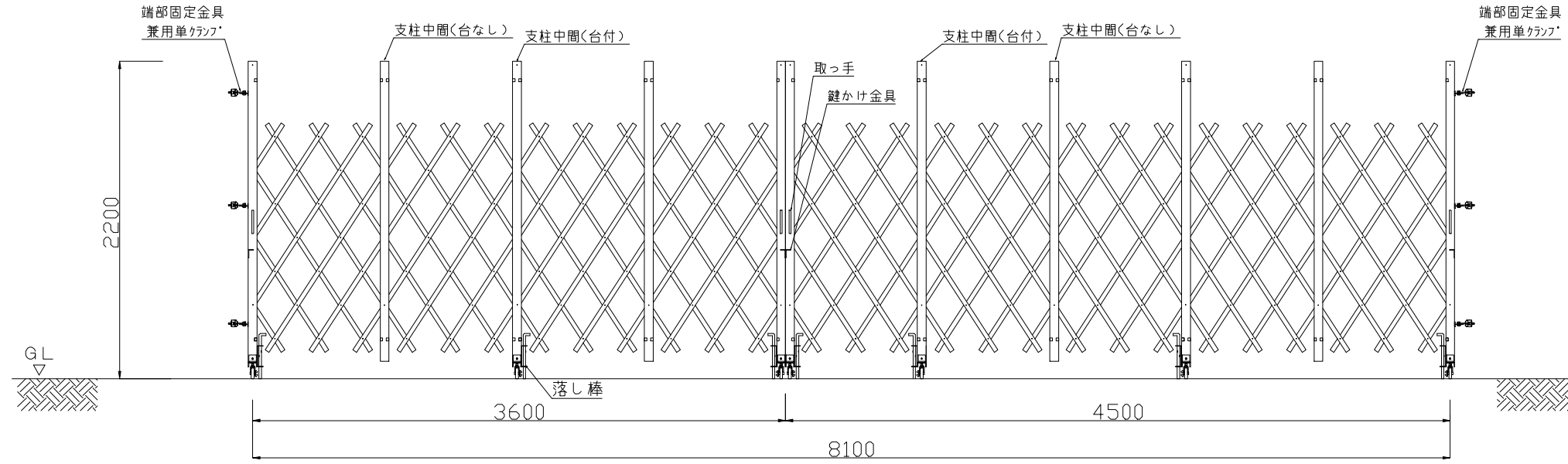
正面図
