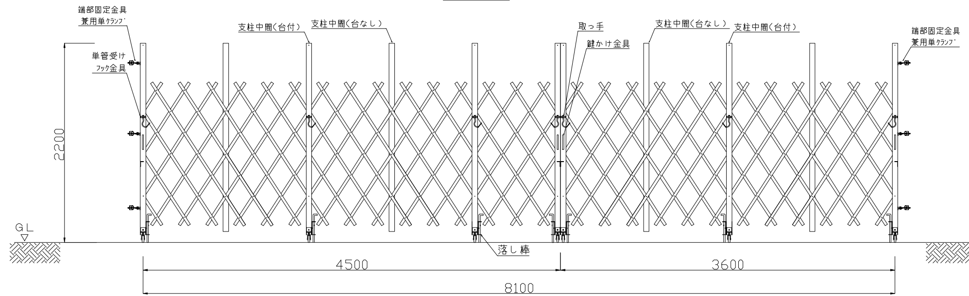
背面図
