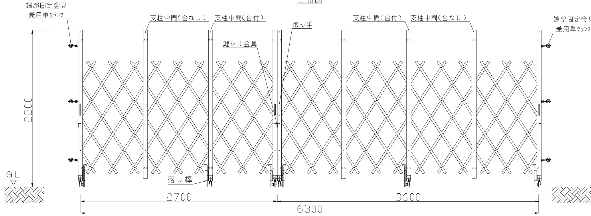
正面図
