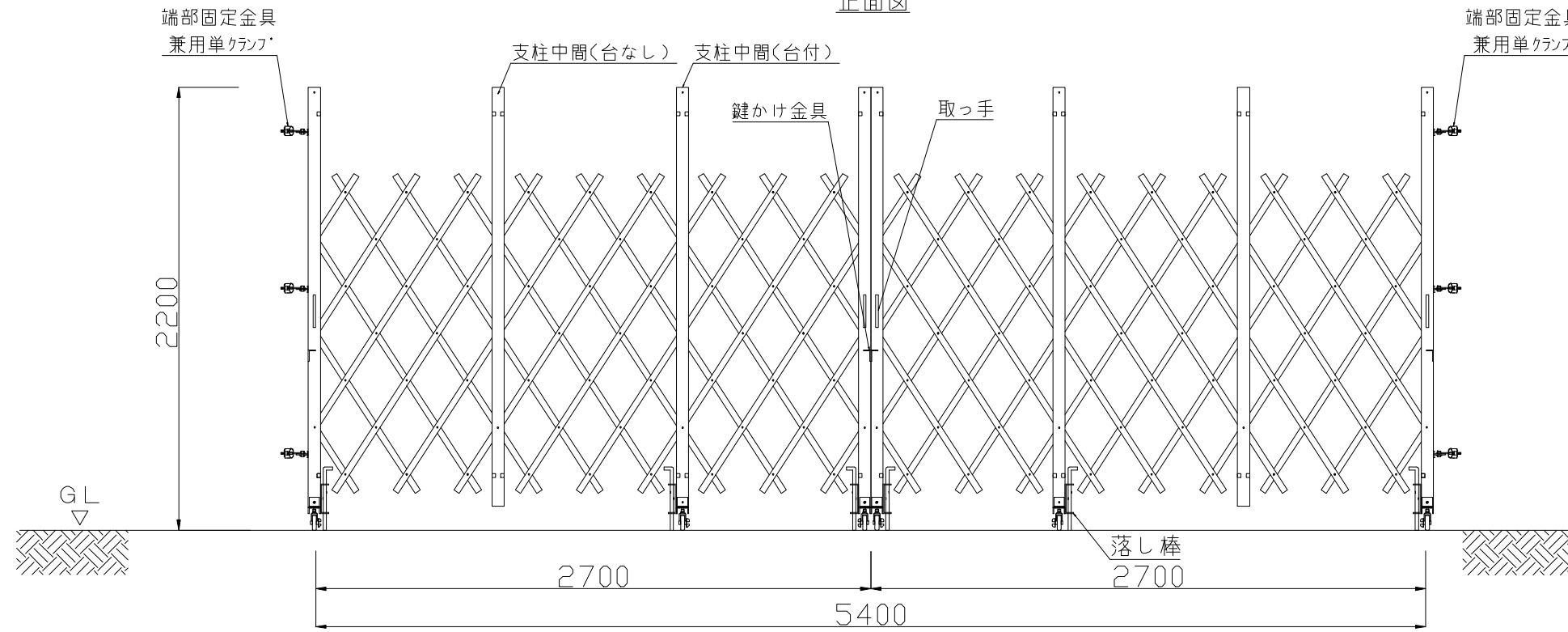
正面図
