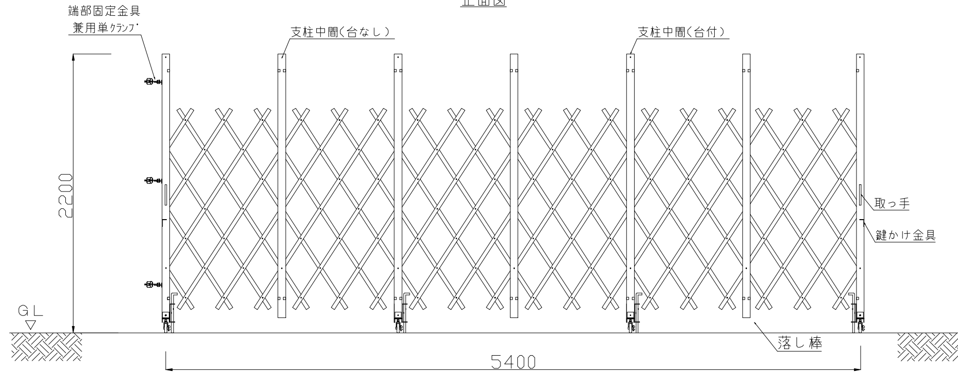
正面図
