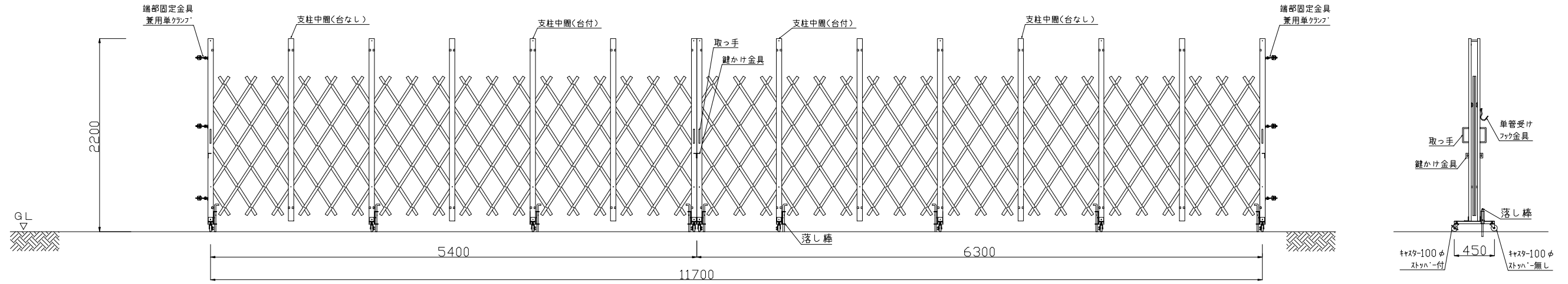
正面図
