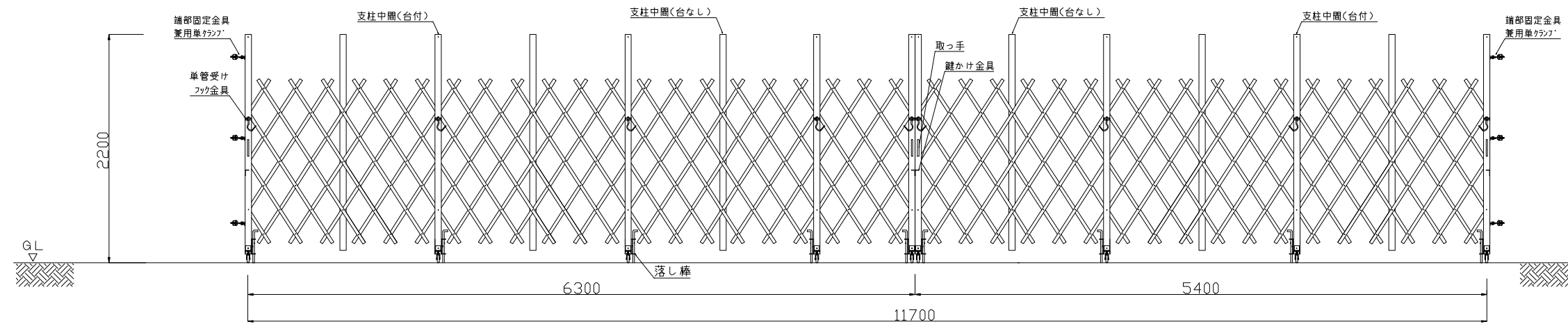
背面図
