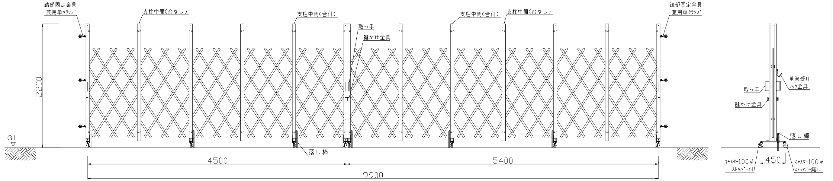
正面図
