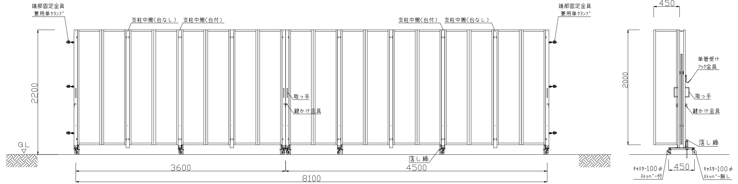
正面図
