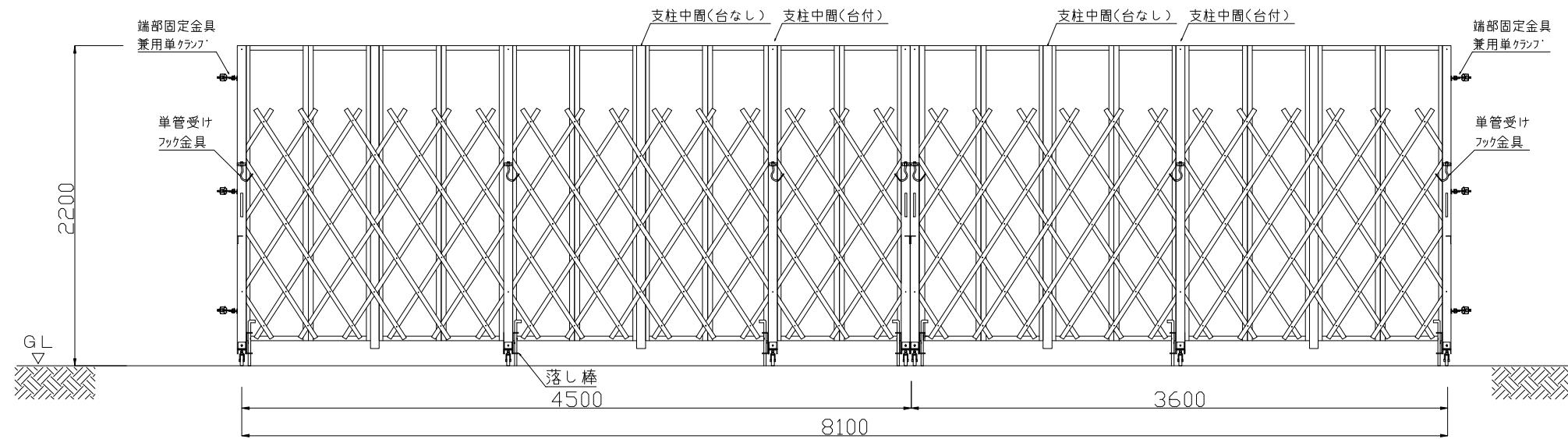
背面図
