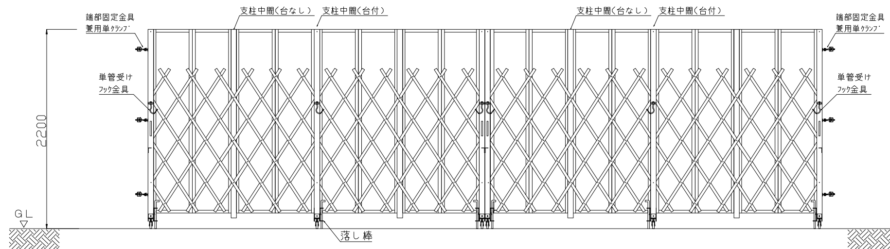
背面図
