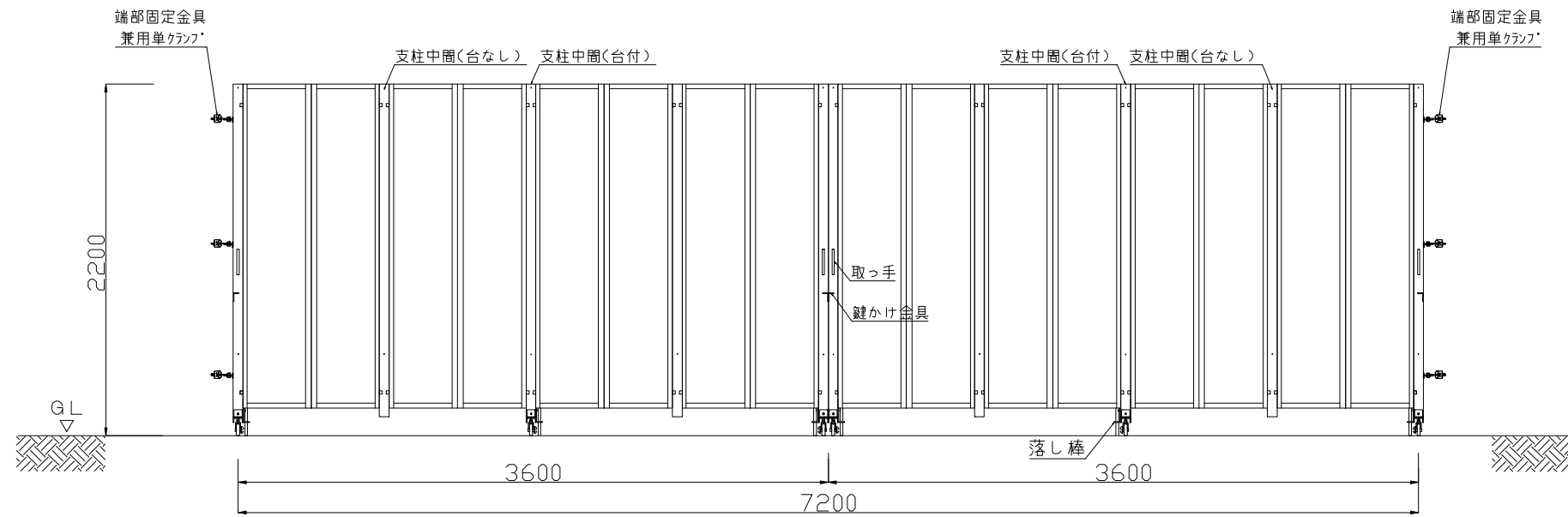
正面図
