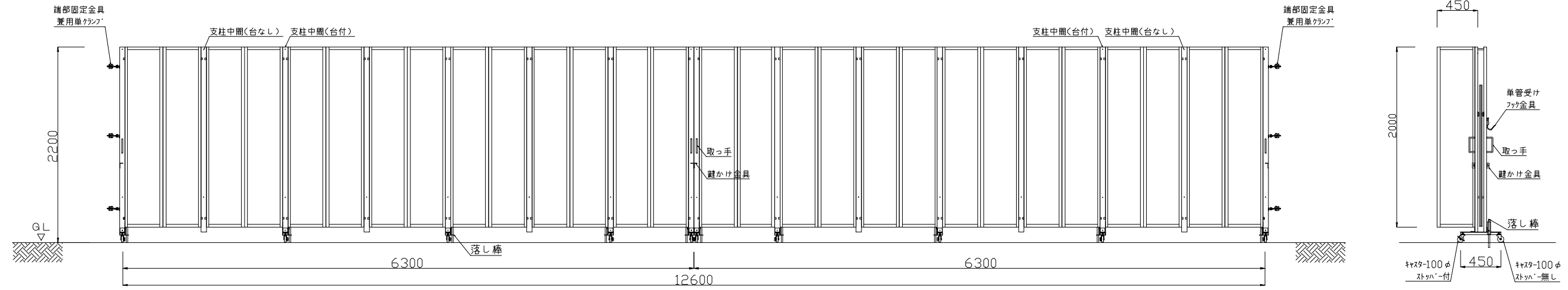
正面図
