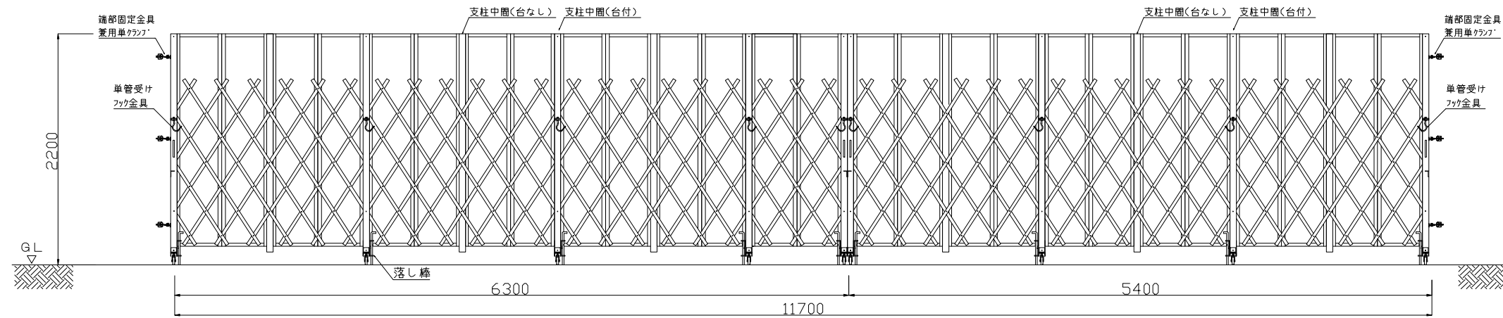
背面図
