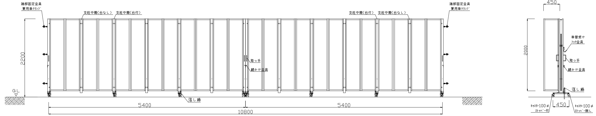
正面図
