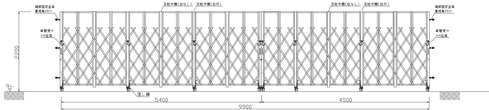
背面図
