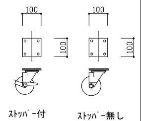
⑥キャスター-100φ (シングル) 詳細図
