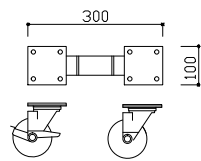
⑥キャスター-100φ (ダブル) 詳細図
