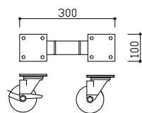
⑥キャスタ-100φ (ダブル) 詳細図
