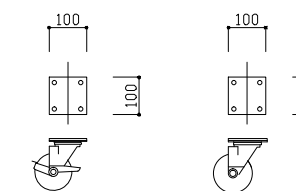
⑥キャスタ-100φ (シングル) 詳細図
