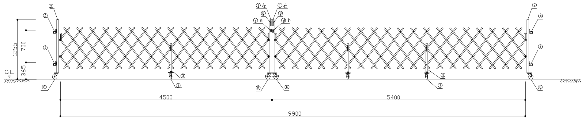
正面図
