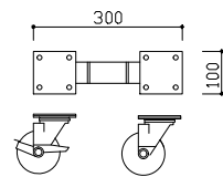
⑦キャスター100φ(ダブル) 詳細図
